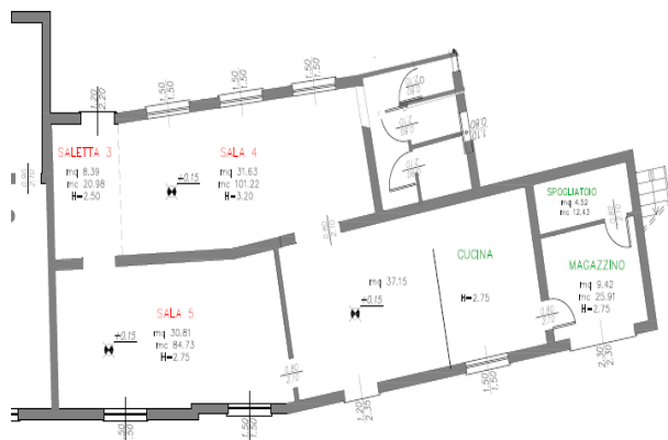
PIANTA PIANO TERRA 1:100
