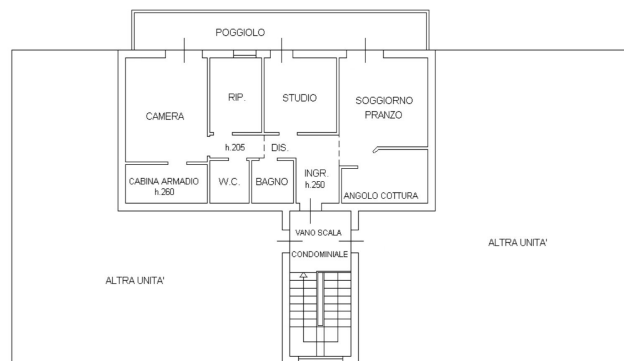
PIANTA PIANO PRIMO H=2.75
